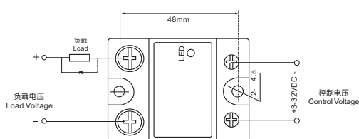
LRSSR - DD接线图
