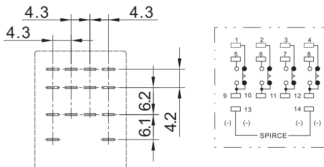
LH3Y L43Y4 接线图
