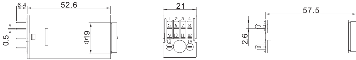
LH3Y L43Y 安装尺寸
