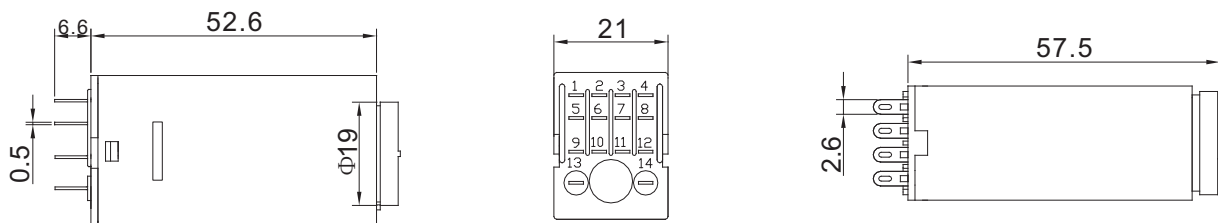
LH3Y L43Y4 安装尺寸
