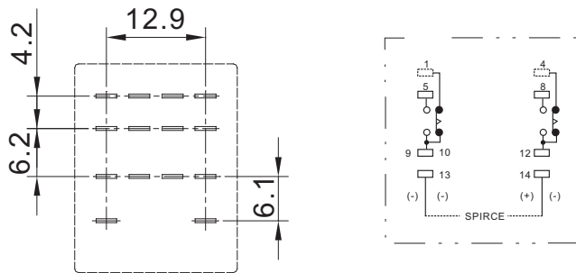
LH3Y L43Y 接线图
